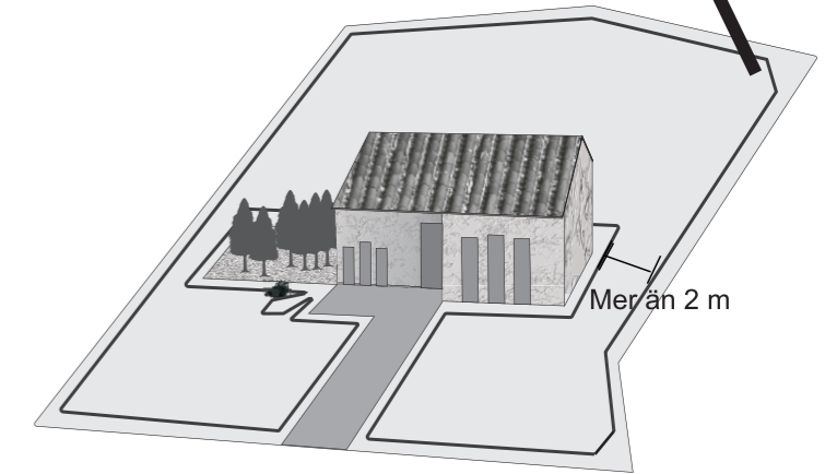
Korrekt hörninstallation
